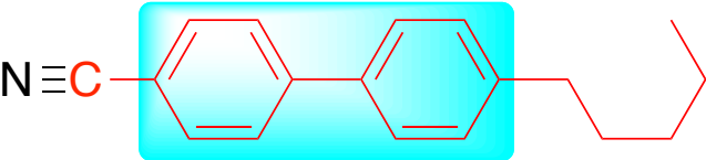
5-CB(液晶)
